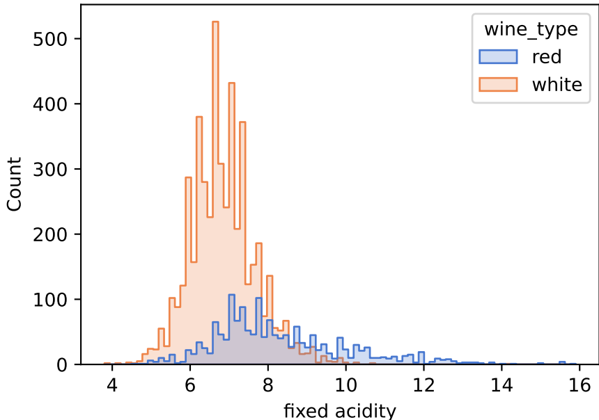
Histograma Incondicional (Bimodalidade) - fixed acidity
